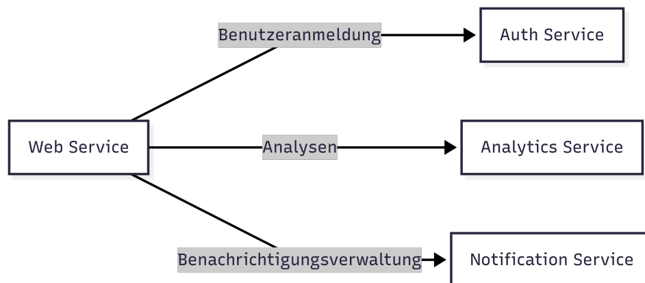
Bild 11: Web Service Interaktionen
