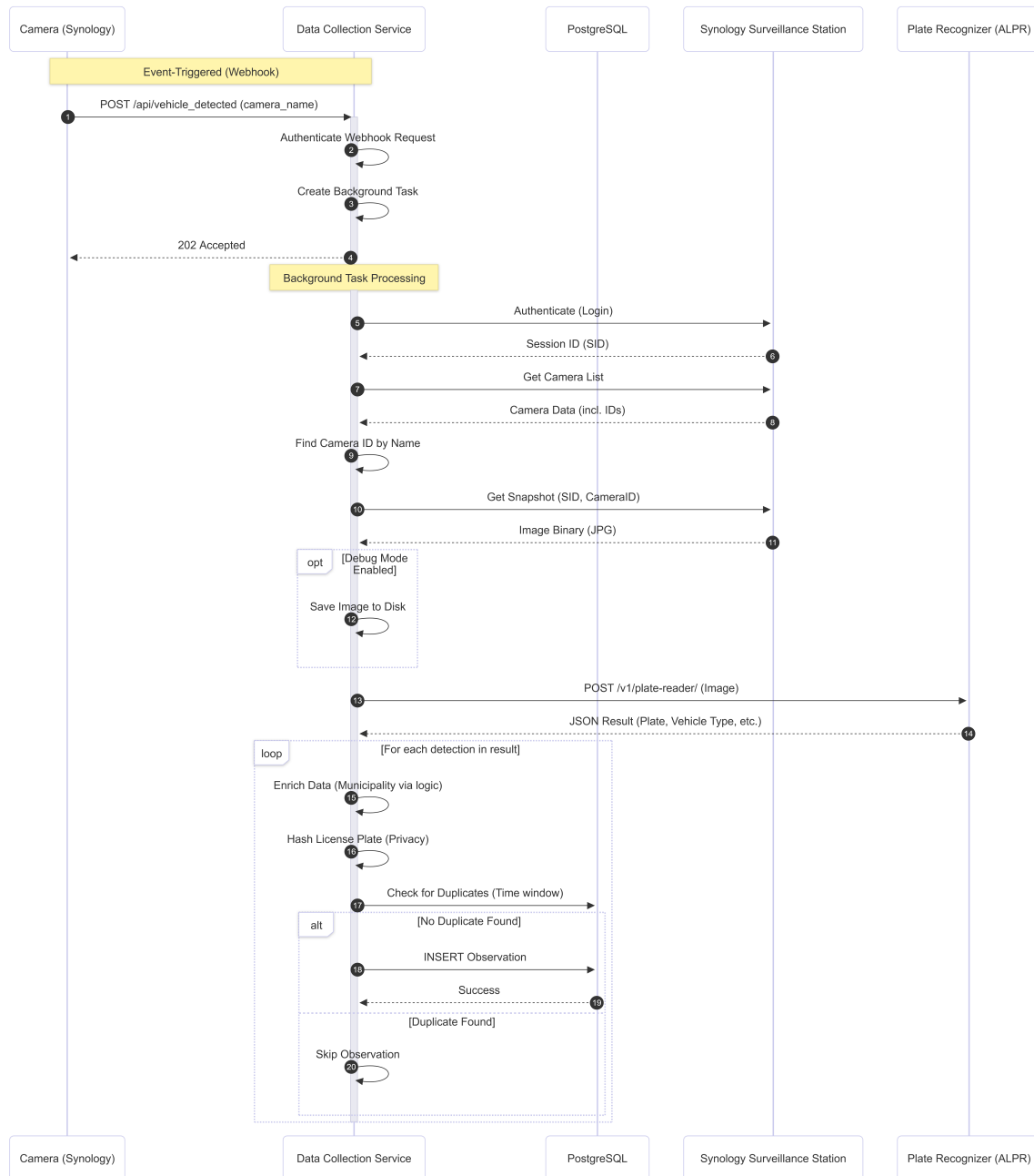
Bild 20: Data Collection Flow
