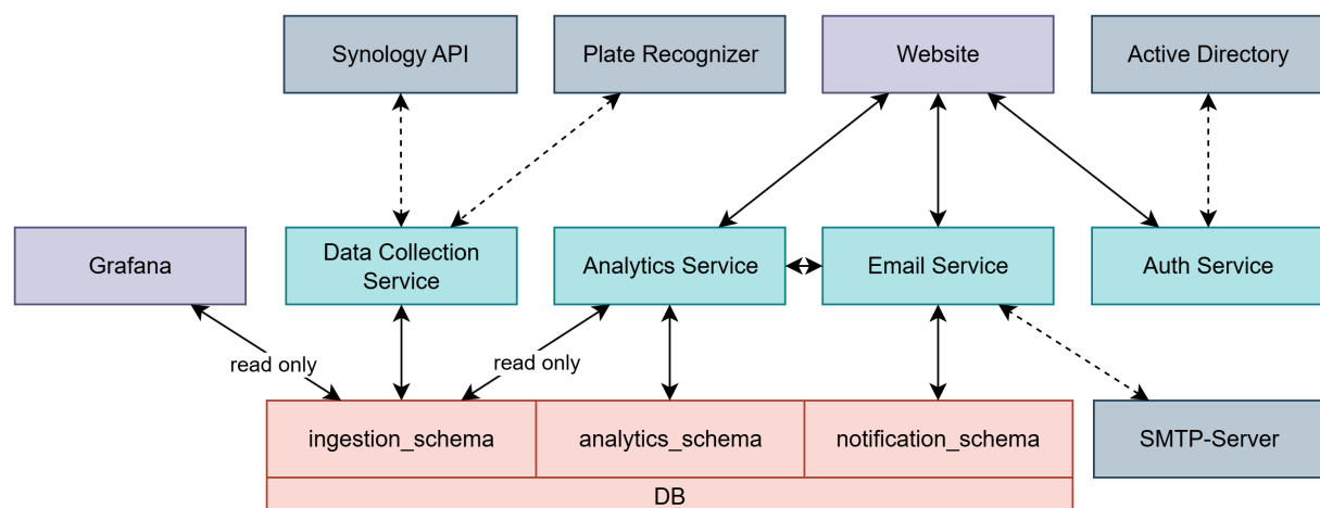
Bild 6: Architektur-Diagramm
