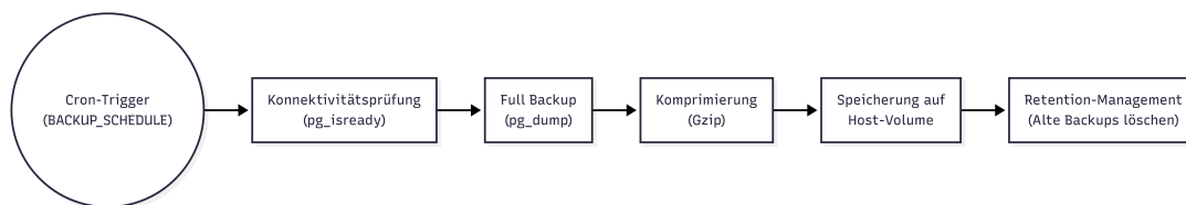
Bild 22: Backup Flow
