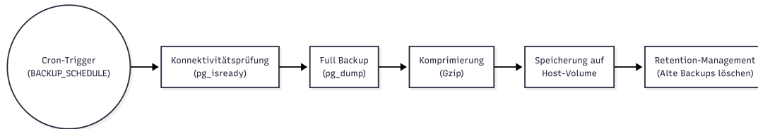
Bild 23: Backup Flow
