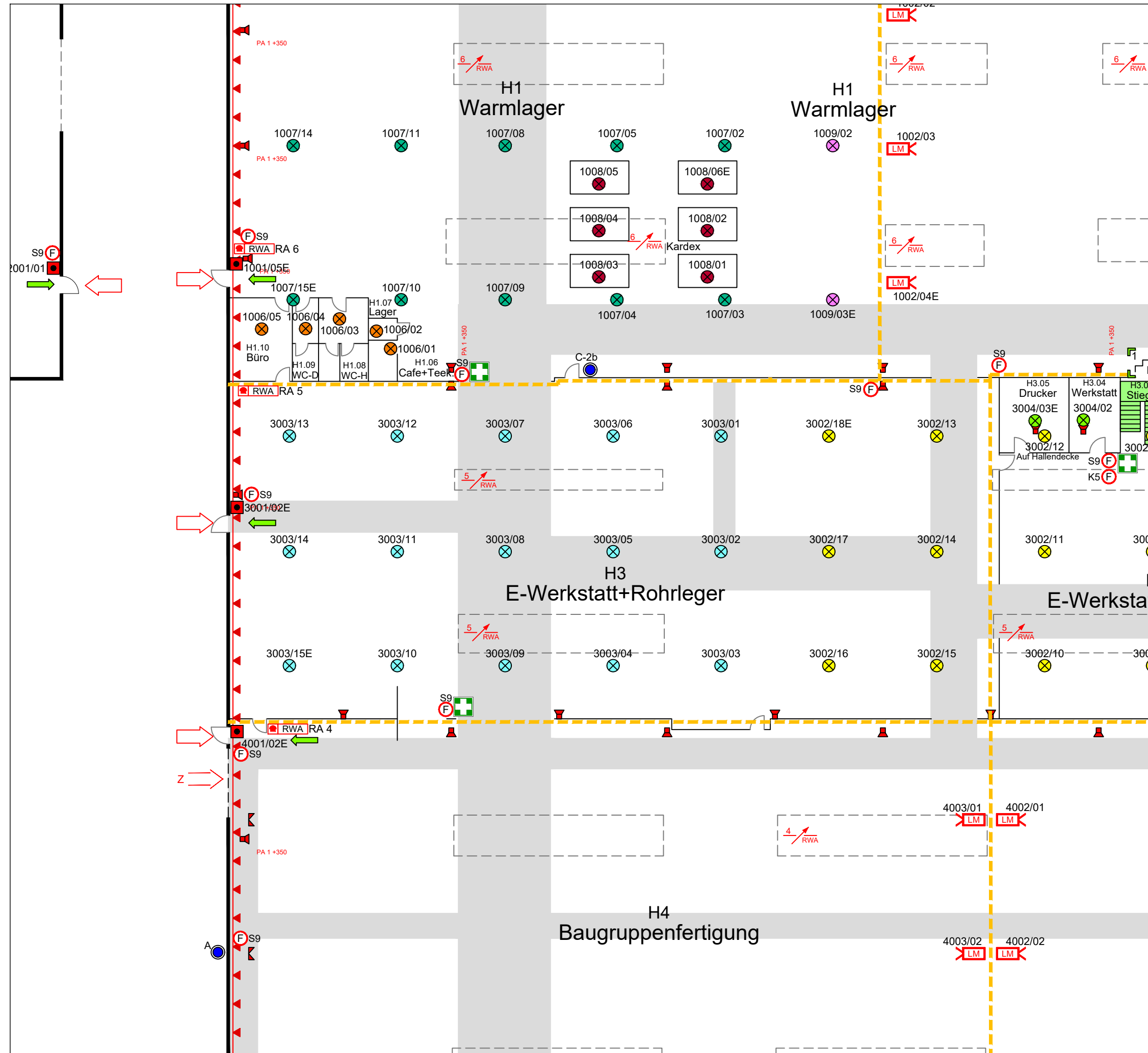
Anschlussplan 16
