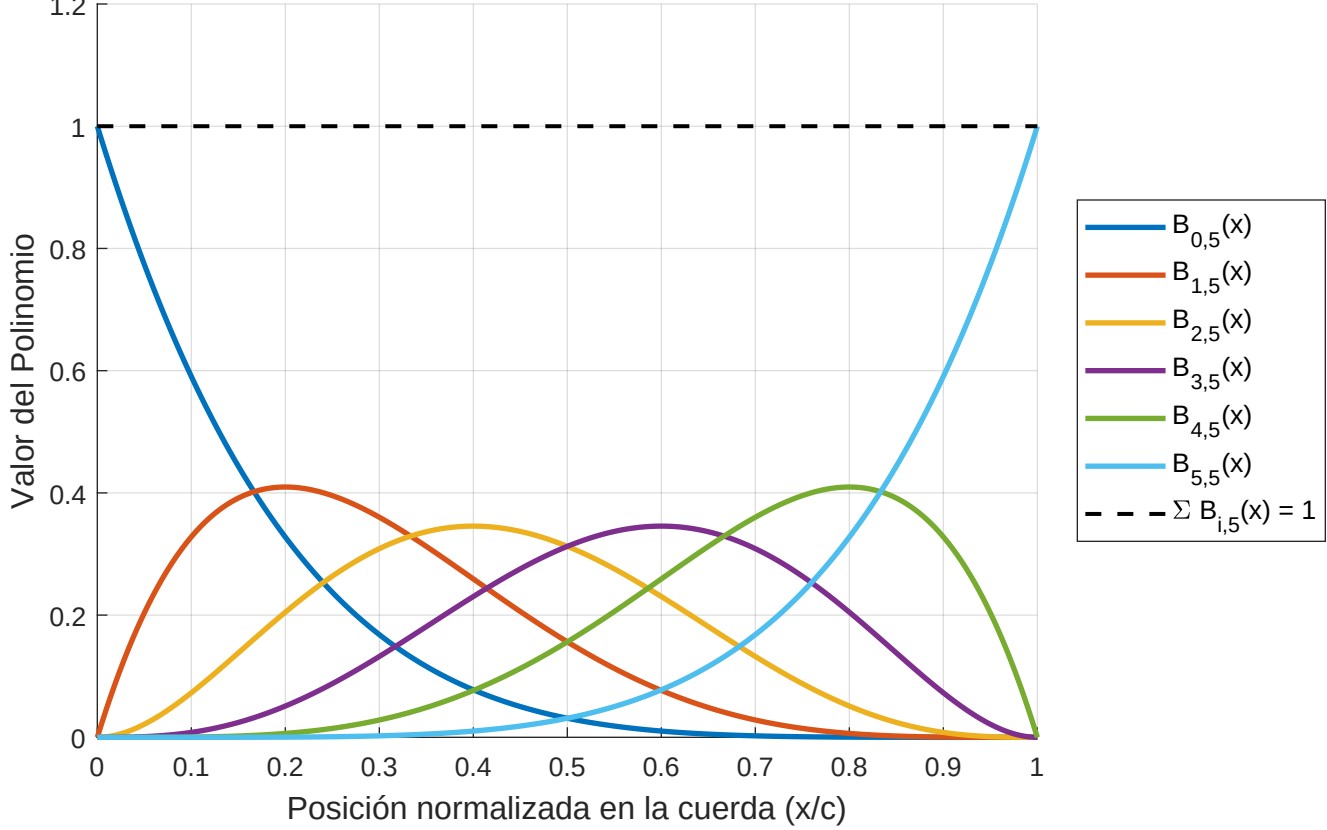
Polinómios de Bernstein de Grado 5 (Base CST)
