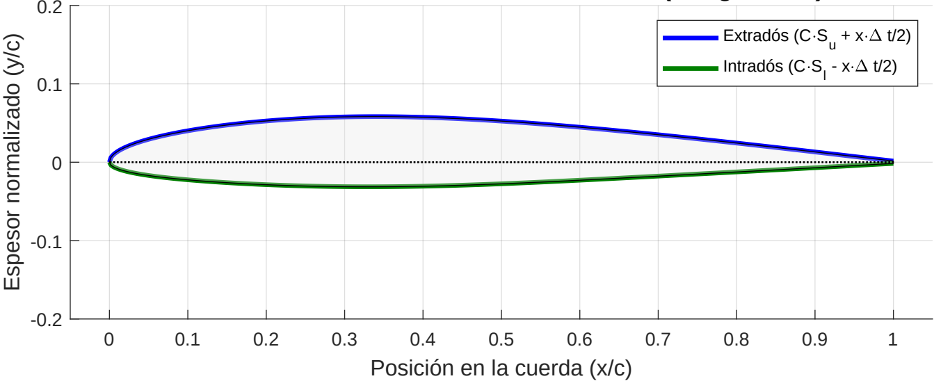
Perfil Alar Reconstruido mediante CST (Selig S3021)
