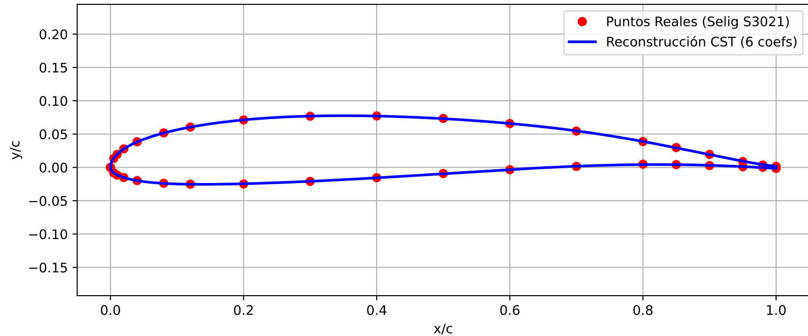
Comparación: Perfil Real vs Reconstrucción CST
