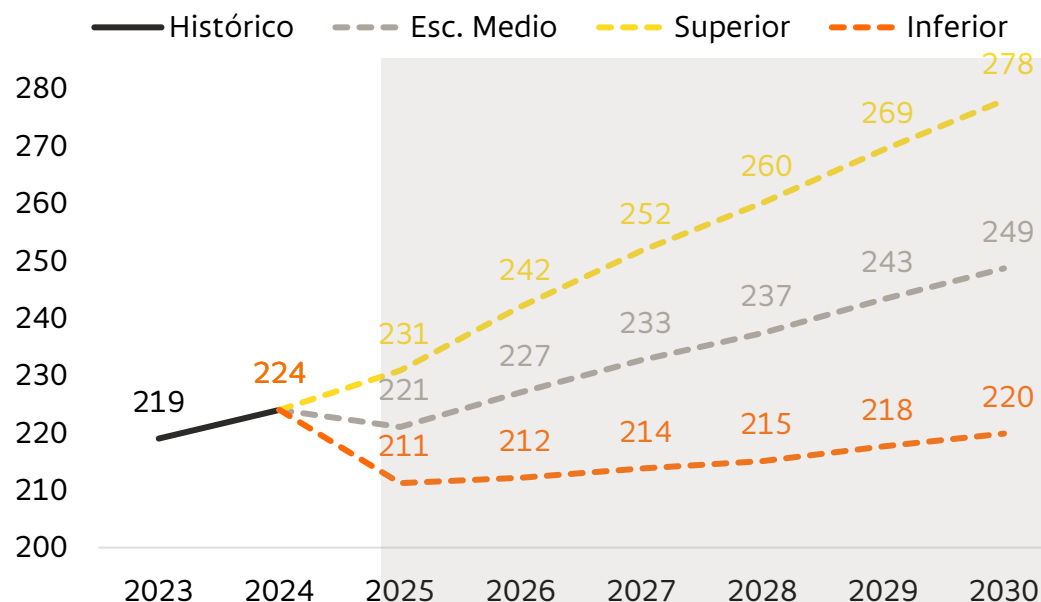
Proyección de demanda de energía SIN (GWh-día)
