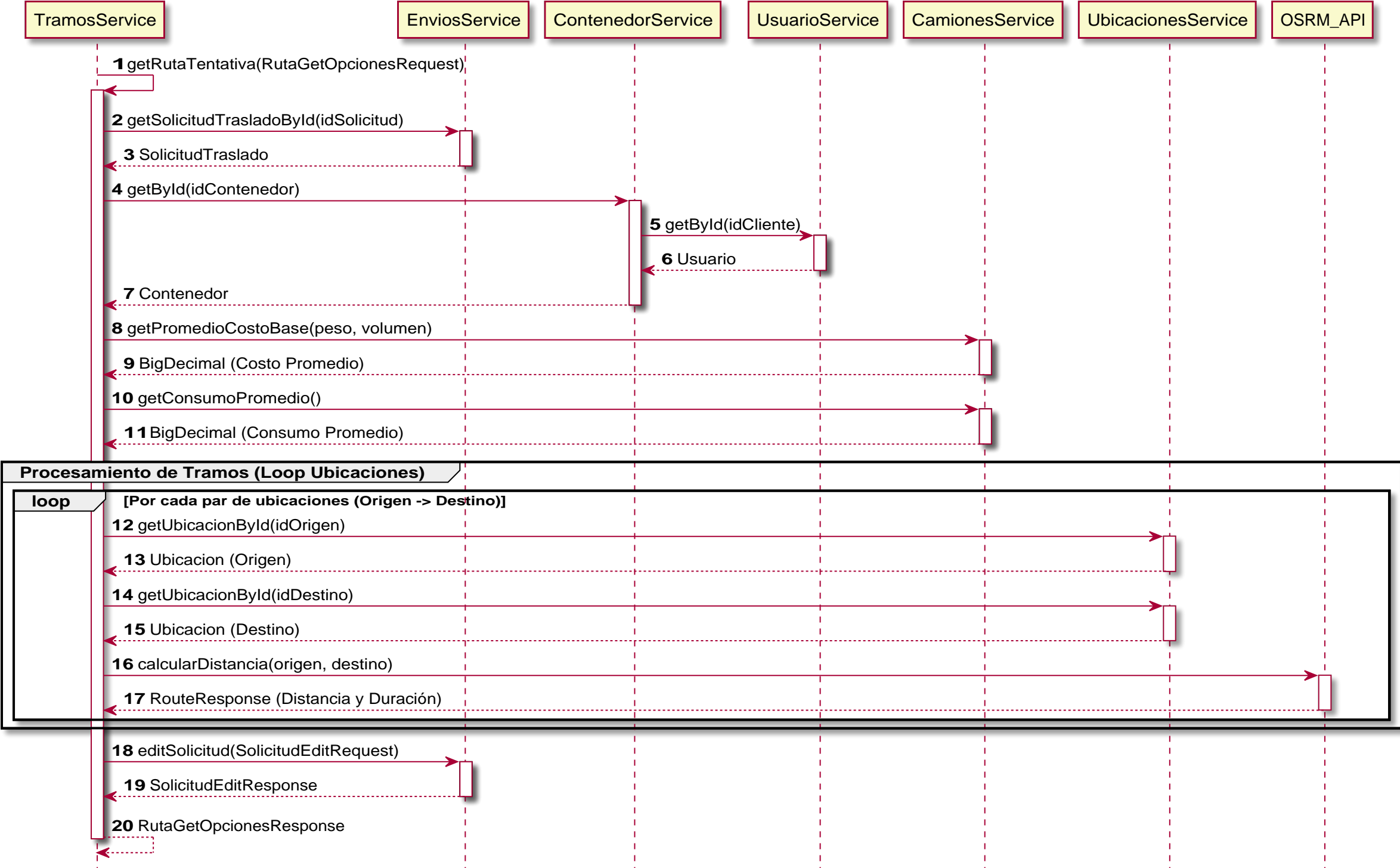
Diagrama de Secuencia: Generar Ruta Tentativa (Interacción Microservicios)
