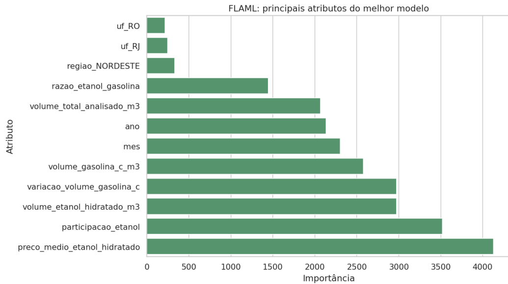
Figura 2: FLAML: principais atributos do melhor modelo selecionado.
