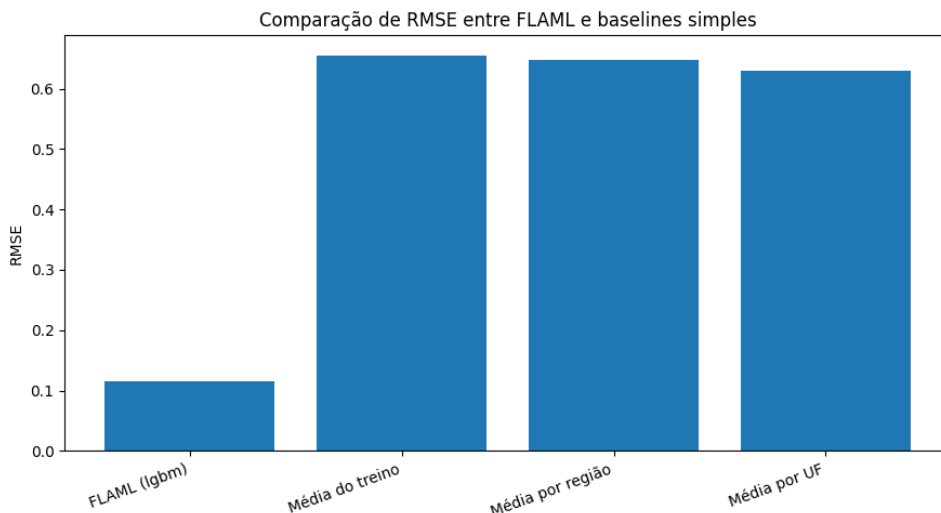
Figura 3: Comparação do RMSE da FLAML com baselines simples.
