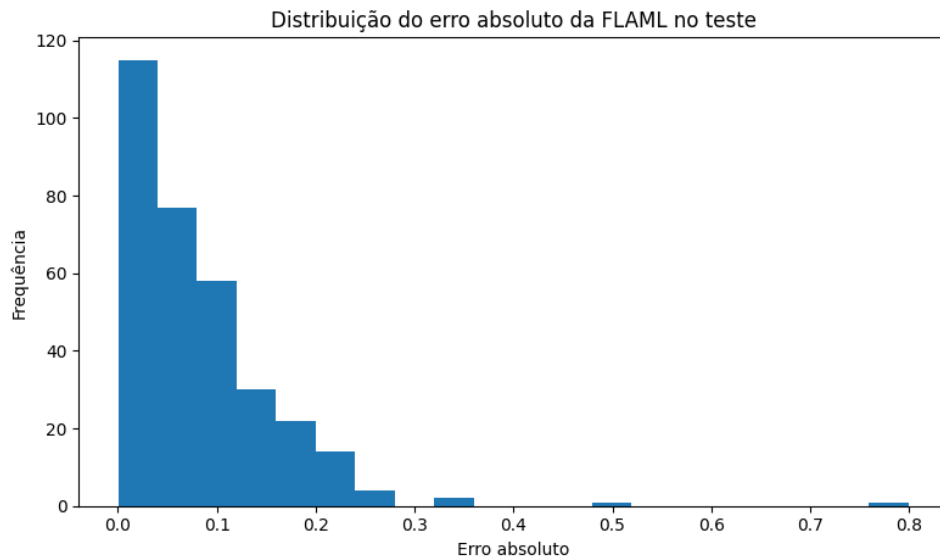
Figura 5: Distribuição dos erros absolutos da FLAML no conjunto de teste.
