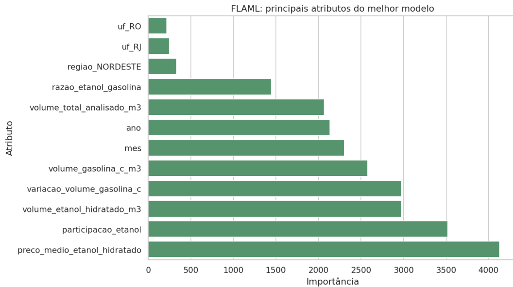
Figura 2: Principais atributos do melhor modelo selecionado pela FLAML.
