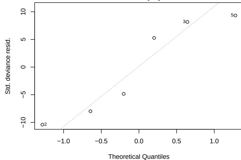
Binomial Normal Q-Q
