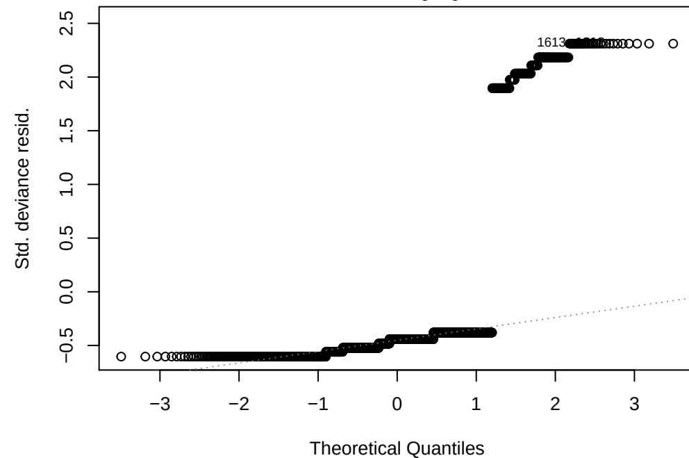
Bernoulli Normal Q-Q
