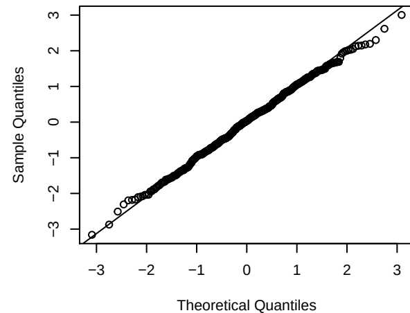
Binomial m=100
