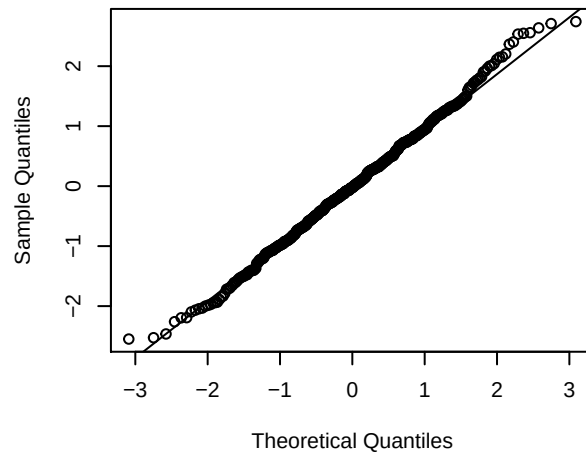
Binomial m=10
