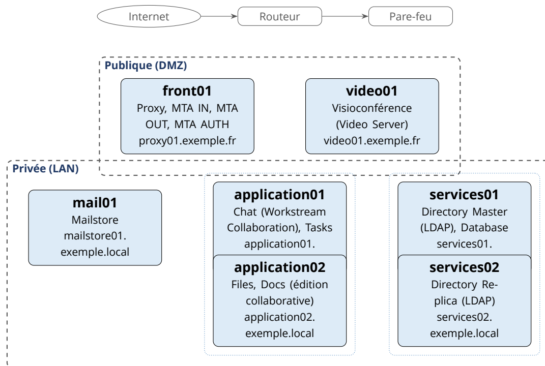
Figure 5.1 – Architecture réseau — Exemple SA (généré depuis client_exemple.yaml )
