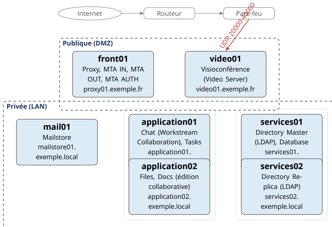
Figure 5.5 – Flux — UDP (visioconférence / RTP)
