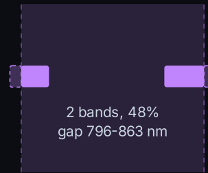
B8 780-886 nm
