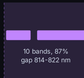
B8 780-886 nm
