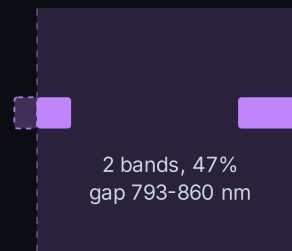
B8 780-886 nm
