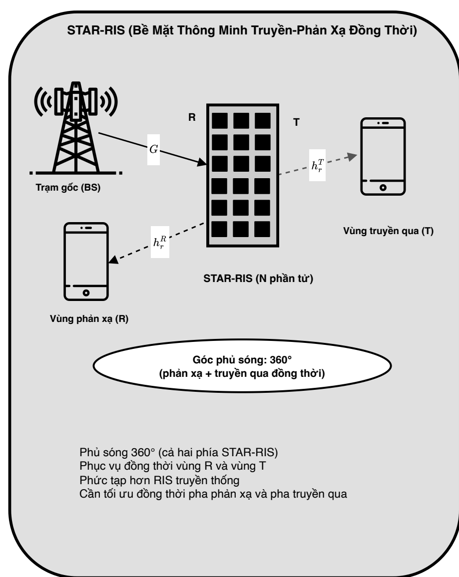
Hình 1.4 – So Sánh RIS Truyền Thống và STAR-RIS
