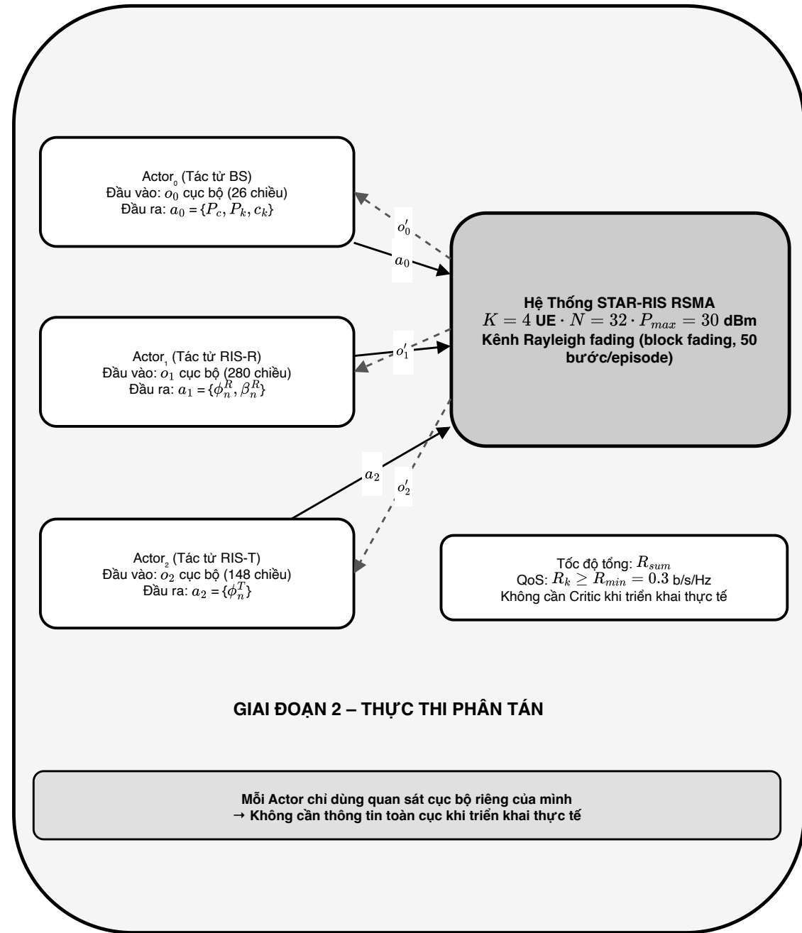
Hình 1.6 – Kiến Trúc MADDPG: Huấn Luyện Tập Trung – Thực Thi Phân Tán (CTDE)
