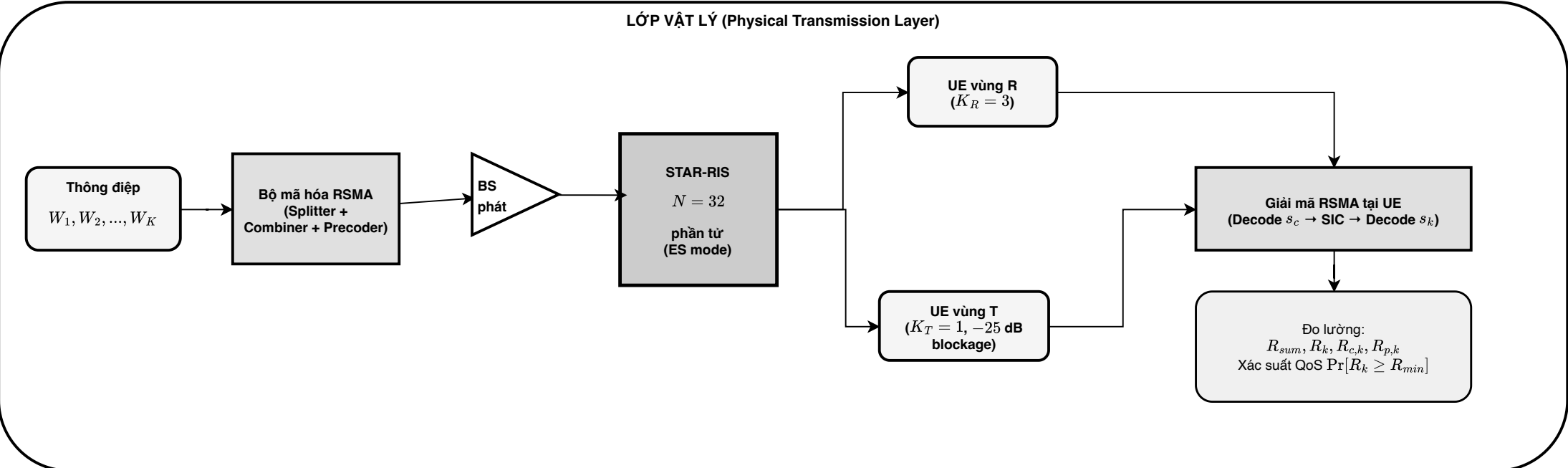
Hình 2.7 – Sơ đồ tổng quan luồng hoạt động hệ thống STAR-RIS RSMA MADDPG
