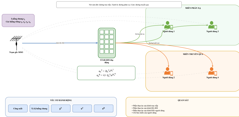
Hình 3.1. Mô hình hệ thống SISO STAR-RIS hỗ trợ RSMA
