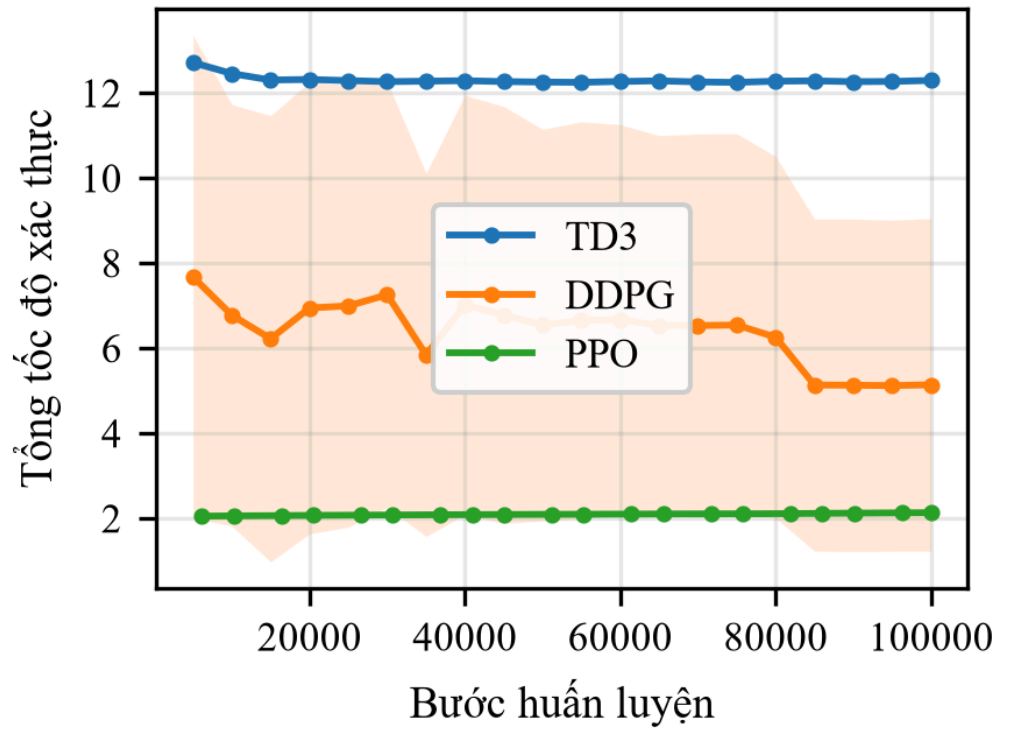
Sum-rate xác thực tại N = 128
