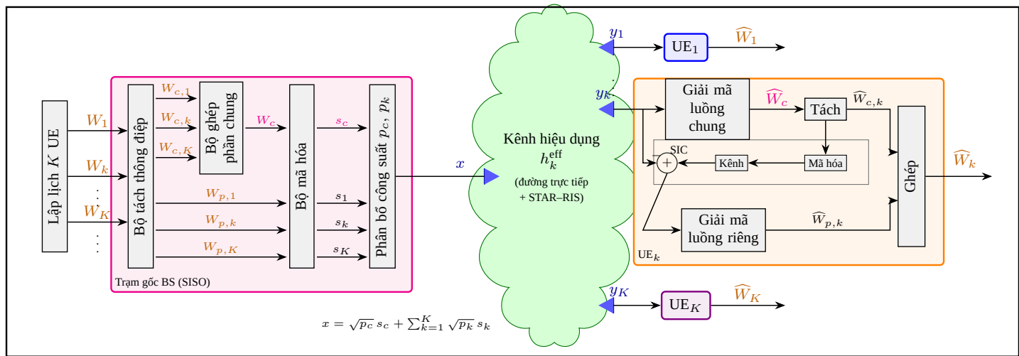
Hình 2.3: Kiến trúc thu-phát RSMA một lớp cho K UE trong hệ SISO
