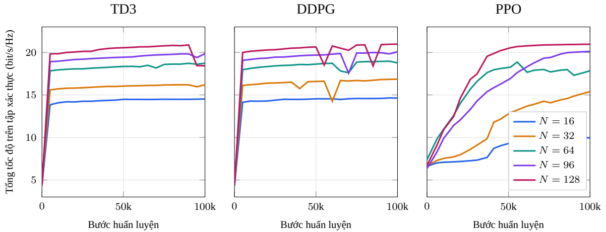
Hình 4.1: Diễn biến tổng tốc độ trên tập xác thực trong quá trình huấn luyện
