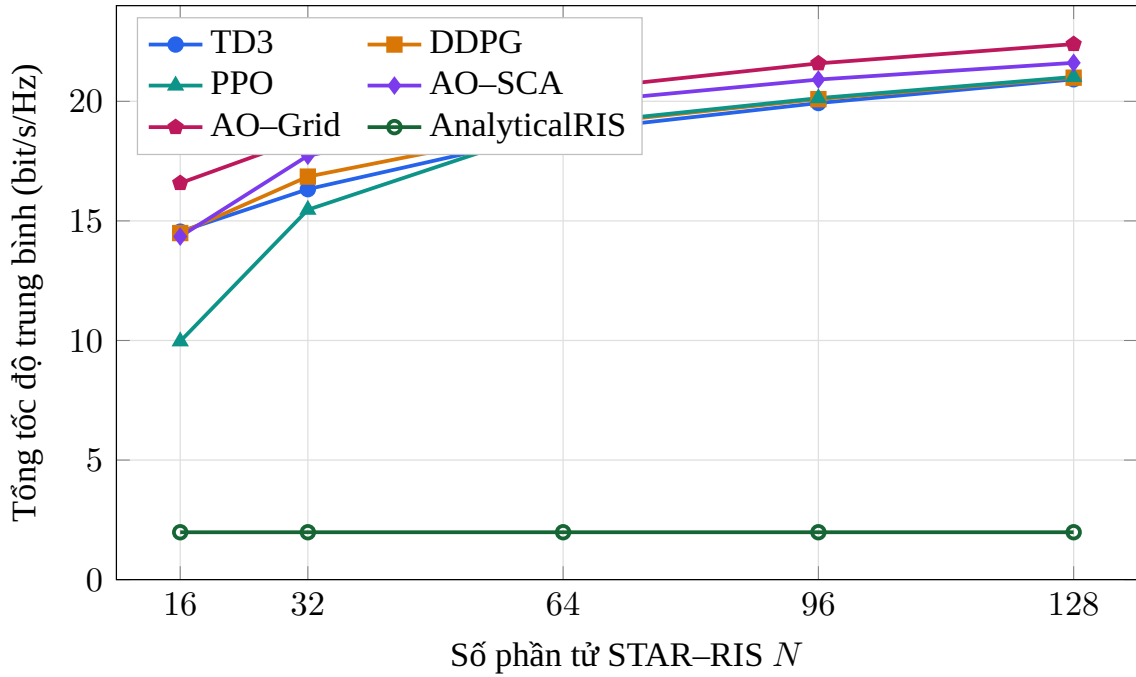
Hình 4.2: Tổng tốc độ của sáu phương pháp theo số phần tử STAR-RIS
