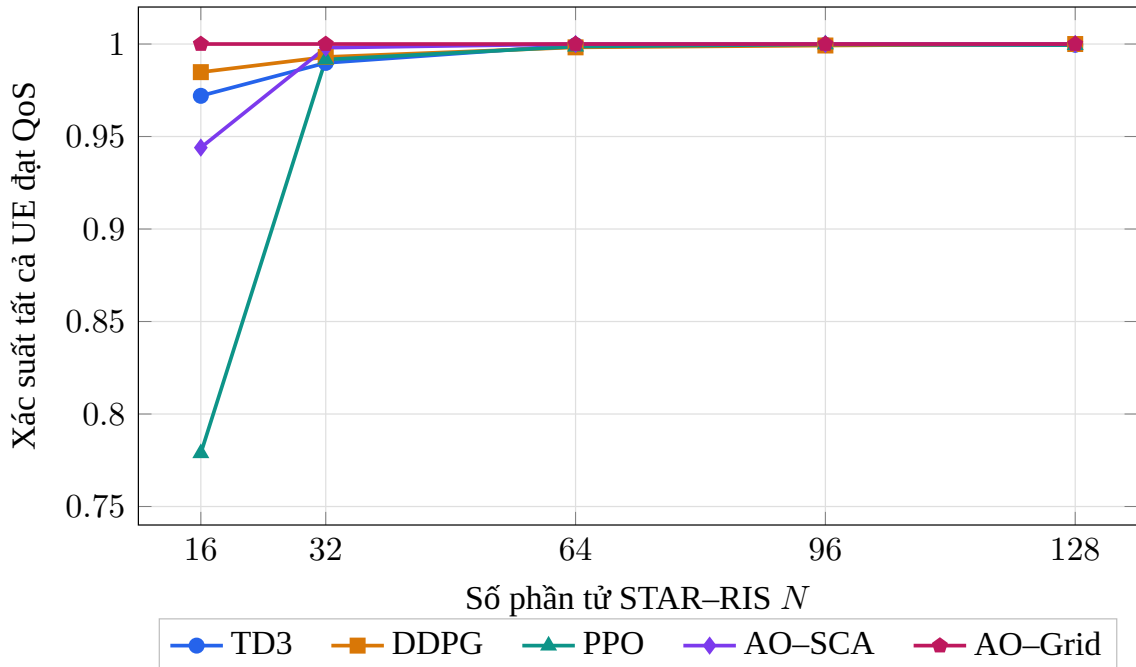
Hình 4.3: Xác suất tất cả UE đạt QoS của các phương pháp có chất lượng cạnh tranh
