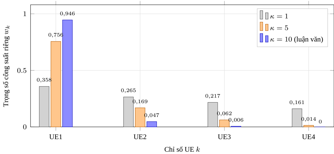
Hình 3.3: Ảnh hưởng của hệ số độ sắc \kappa đến phân bố công suất luồng riêng
