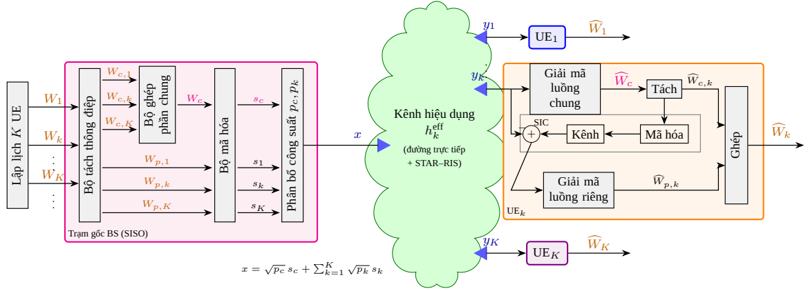
Hình 2.2: Kiến trúc thu–phát RSMA một lớp cho K UE trong hệ SISO
