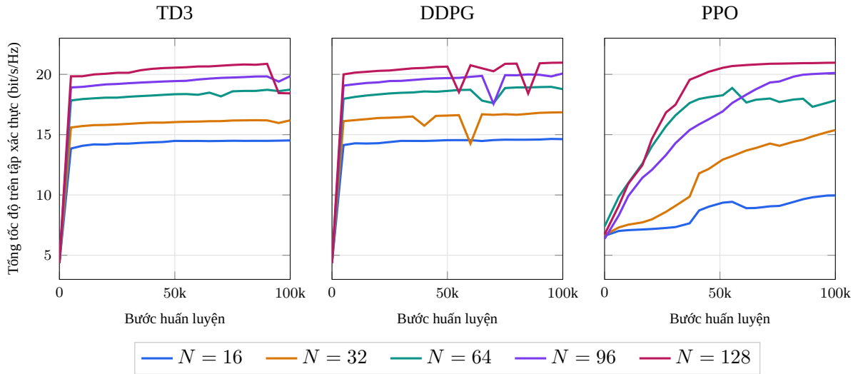
Hình 4.1: Diễn biến tổng tốc độ trên tập xác thực trong quá trình huấn luyện
