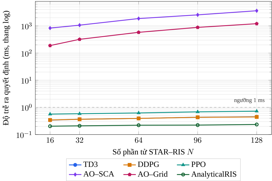
Hình 4.4: Độ trễ ra quyết định khi số phần tử STAR-RIS tăng
