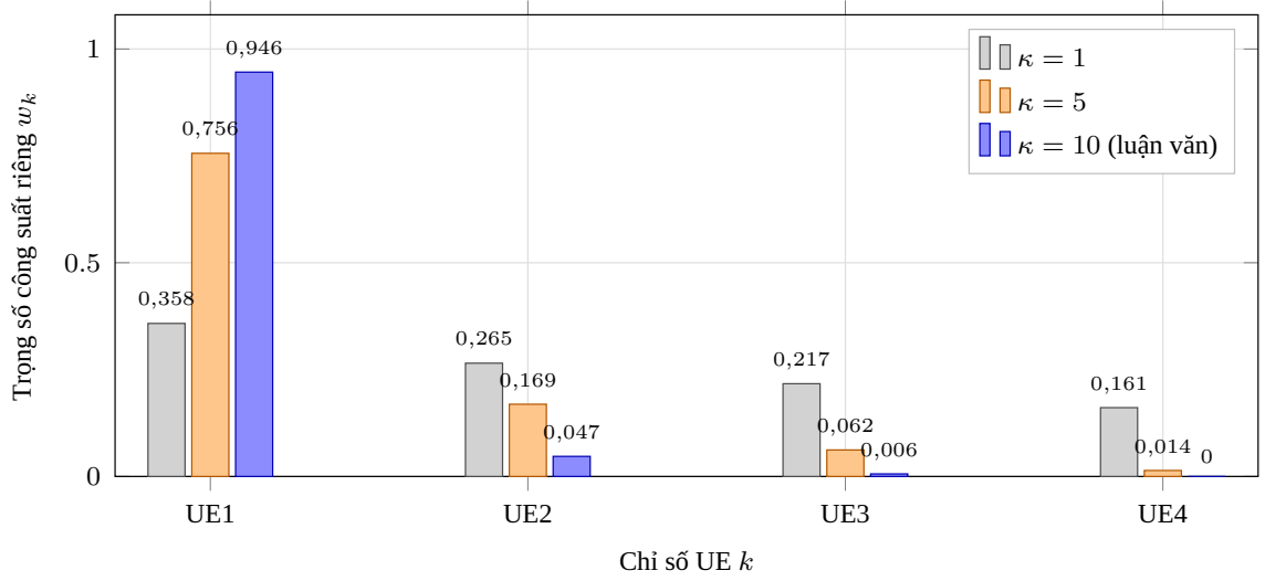
Hình 3.3: Ảnh hưởng của hệ số độ sắc \kappa đến phân bố công suất luồng riêng
