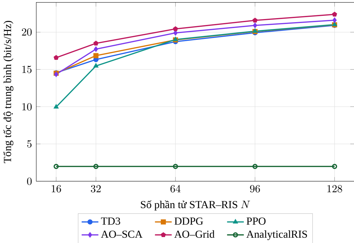
Hình 4.2: Tổng tốc độ của sáu phương pháp theo số phần tử STAR-RIS
