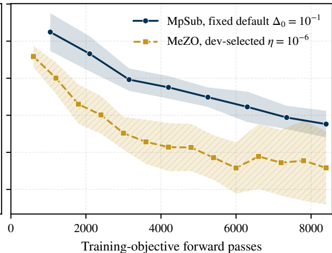
OPT-350M
