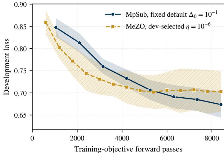
OPT-125M
