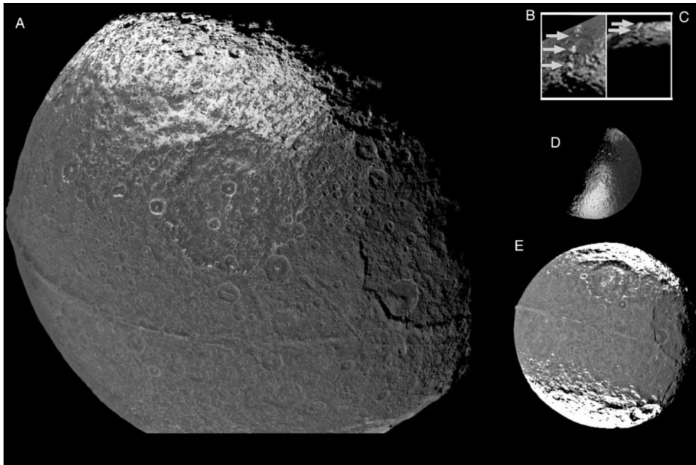
Abbildung 3: Aufnahmen der Saturnmondes Iapetus. Der Bergkamm ist deutlich am Äquator erkennbar. (Porco, 2005: S.1240).
