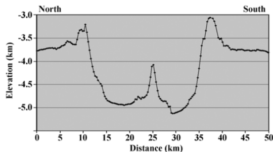
Abbildung 1: Topografisches Profil des Tooting-Kraters, das durch den höchsten Punkt des Zentralbergs verläuft. (Mouginis-Mark, 2012: S.1619).
