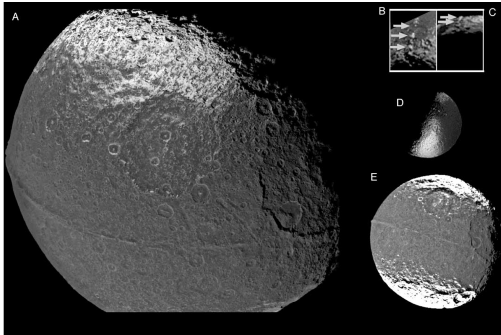
Abbildung 2: Aufnahmen der Saturnmonde Iapetus. Der Bergkamm ist deutlich am Äquator erkennbar. (Porco, 2005: S.1240).
