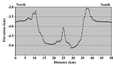
Abbildung 1: Topografisches Profil des Toth-Krater, das durch den höchsten Punkt des Zentralbergs verläuft. Die vertikale Maßstabsverzerrung beträgt \times 10 . Entnommen aus (Mouginis-Mark, 2012: S.1619).
