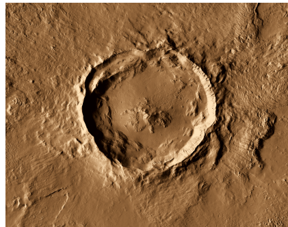
Abbildung 2: Foto des Tooting-Kraters. Ausschnitt von der Aufnahme der THEMIS-Mission der NASA. (NASA, o.J.).
