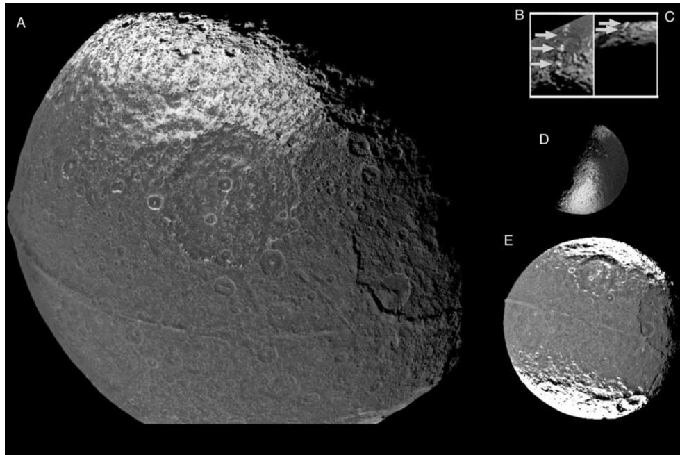
Abbildung 3: Aufnahmen des Saturnmondes Iapetus. Der Bergkamm ist deutlich am Äquator erkennbar. (Porco, 2005: S.1240).
