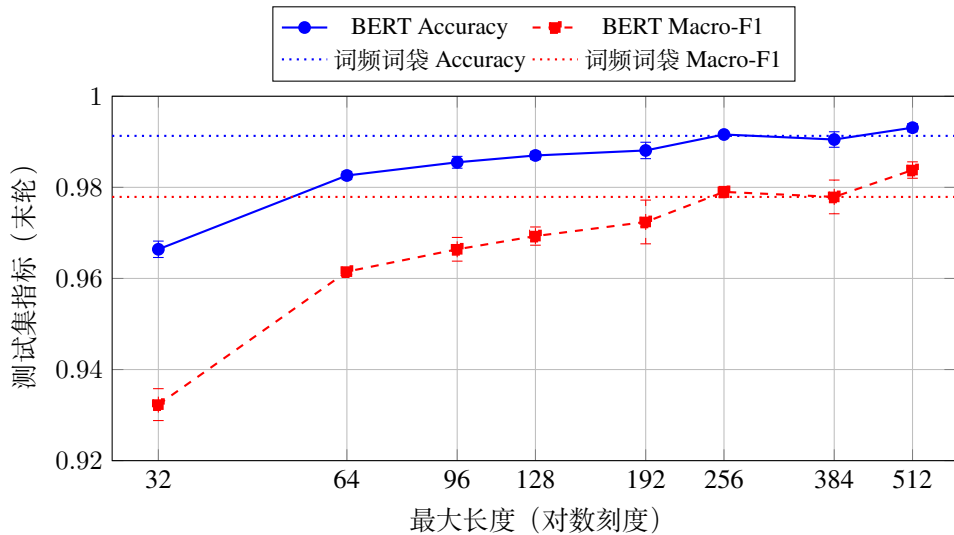
图 5: BERT 测试集指标随最大长度的变化（误差棒为 3 个种子的标准差）。水平点线为词频词袋的结果
