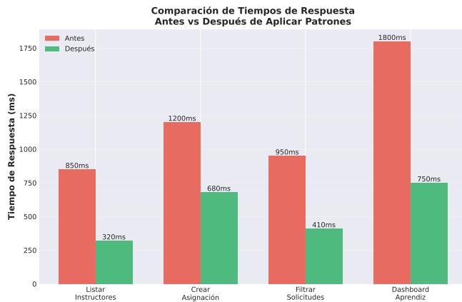
Figura 4: Comparación de tiempos de respuesta antes y después de aplicar patrones
