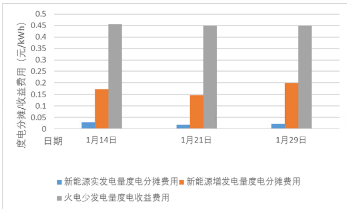
图 1：火电企业与新能源企业收益与分摊
