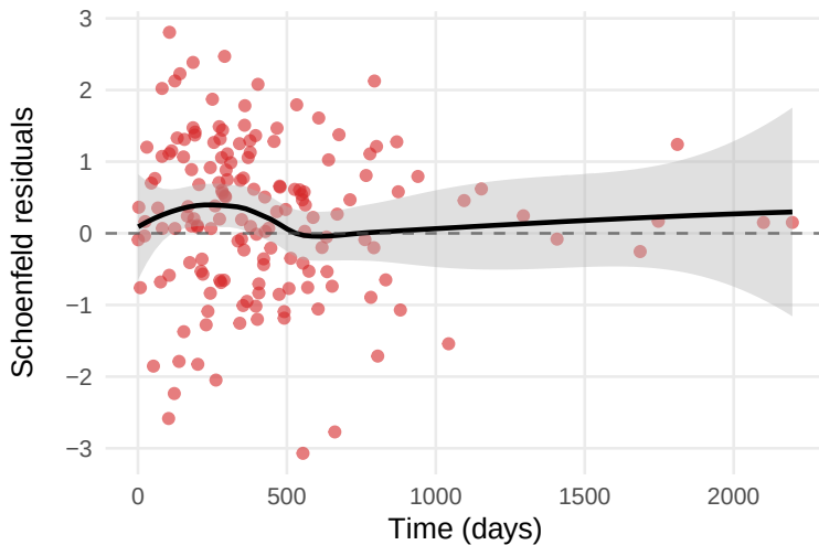
BMP1 (p = 0.0644)
