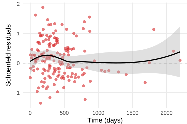
PDGFD (p = 0.741)
