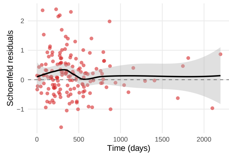
TSPAN18 (p = 0.3141)
