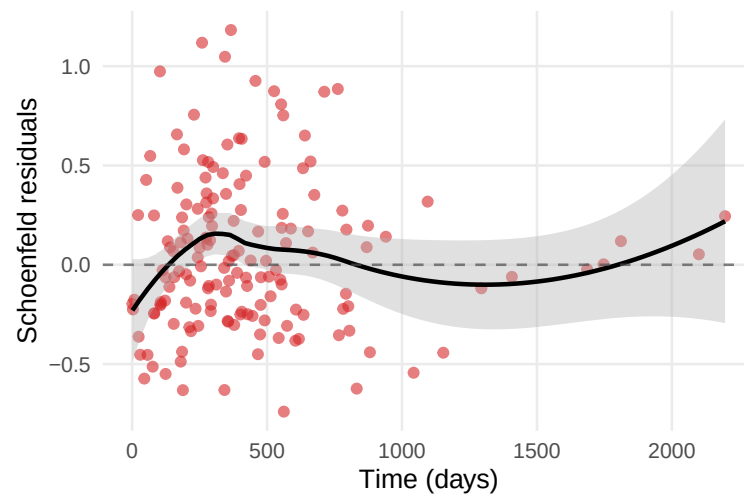
TSPAN7 (p = 0.2722)
