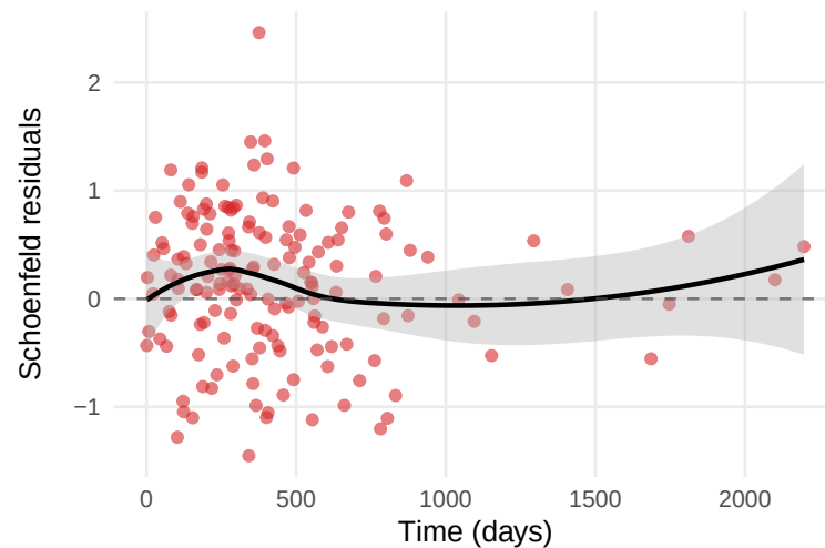
TSPAN5 (p = 0.3628)
