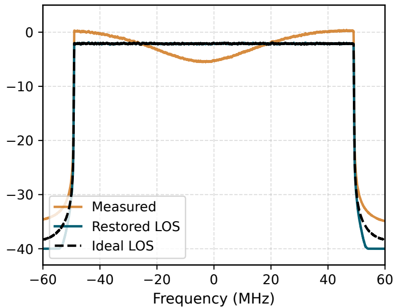
(d) LOS restoration
