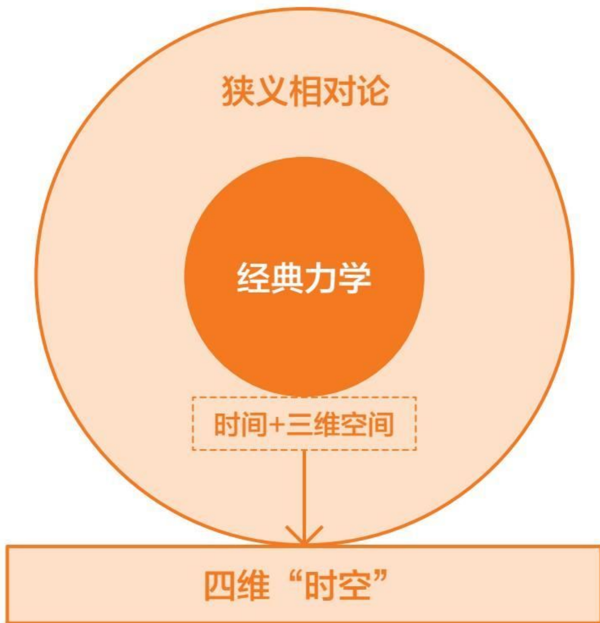
图6-2 从三维空间升级为四维时空
