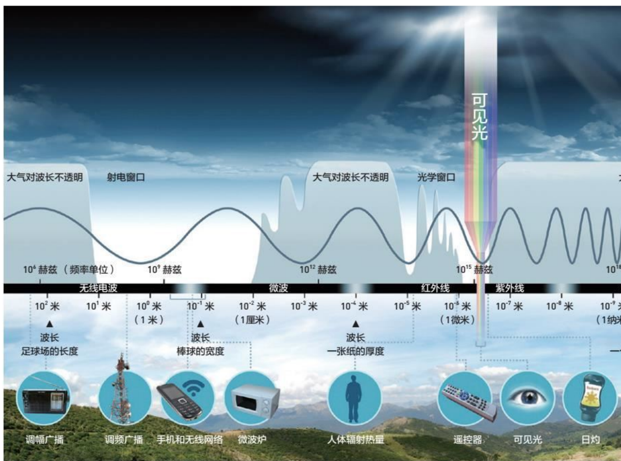
图7-2 人的可见光频段示意图
