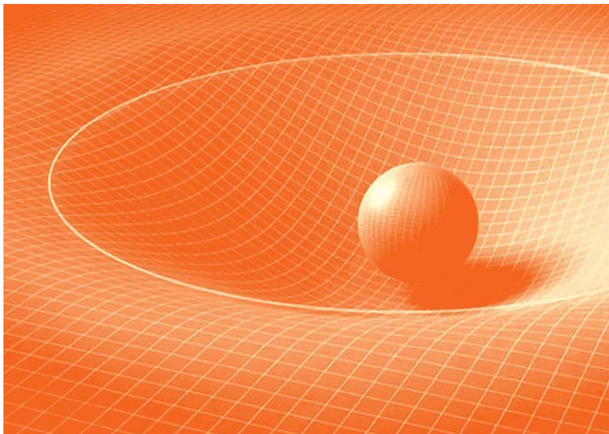
图6-3 弯曲的时空场
