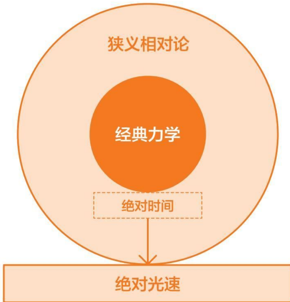
图6-1 从绝对时间升级为绝对光速
