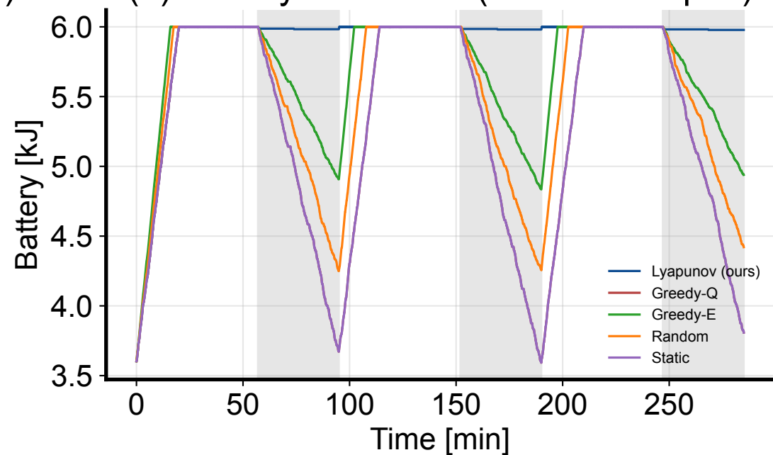
(d) Battery over time (shaded=eclipse)
