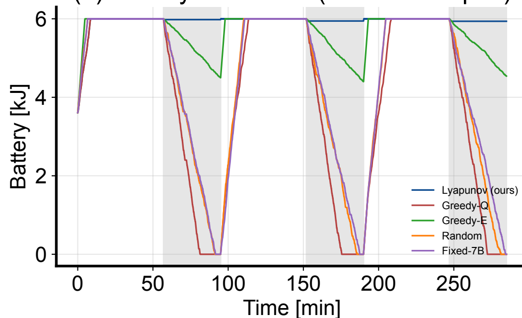
(d) Battery over time (shaded=eclipse)
