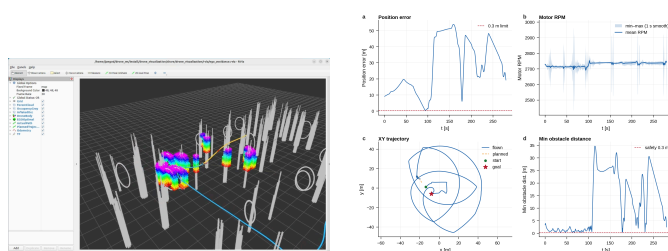
图 11: 场景 4 静态避障: RViz (左) 与评测曲线 (右)
