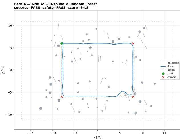
图 16: Path A 森林试次轨迹
