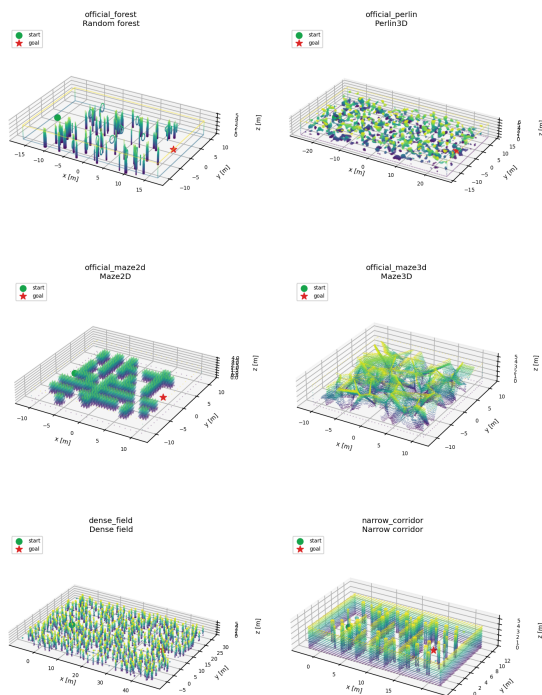
图3: 主要仿真地图三维斜视点云 (三行 \times 两列)。颜色表示高度; 绿点为起点, 红星为目标。
