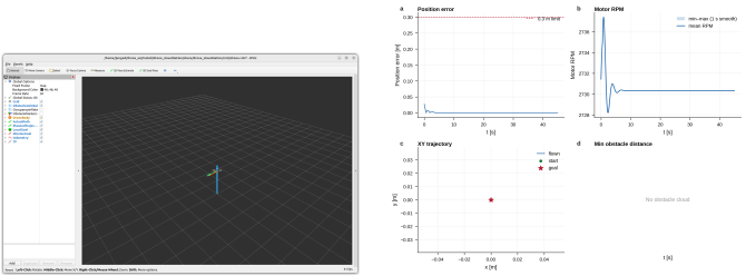
图 8：场景 1 悬停：RViz（左）与评测曲线（右）
