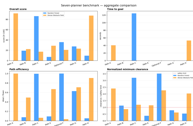
图 14: 规划器对照总览图
