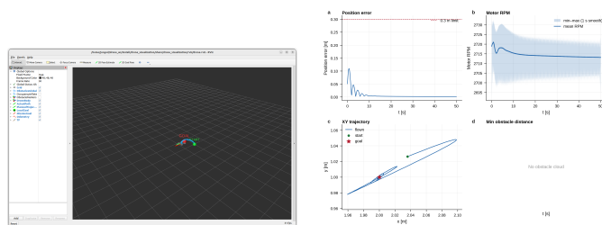
图 9: 场景 2 单目标: RViz (左) 与评测曲线 (右)
