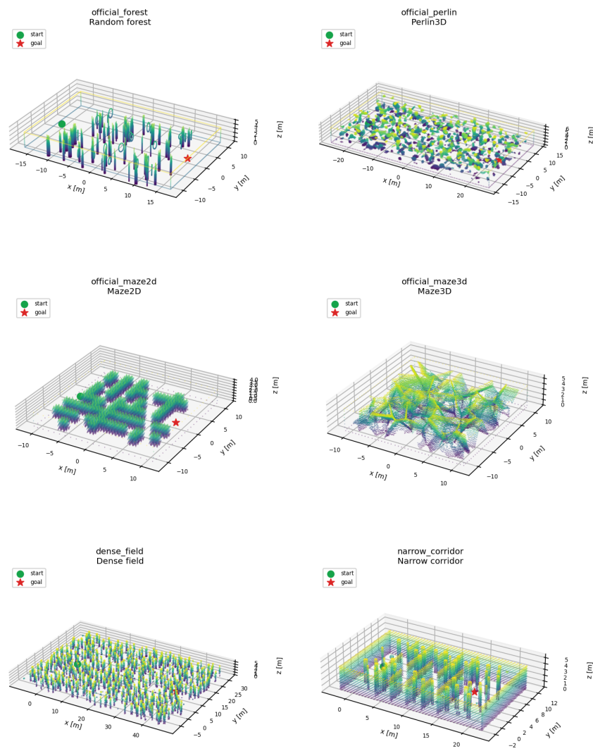
图 3：主要仿真地图三维斜视点云（三行 × 两列）。颜色表示高度；绿点为起点，红星为目标。
