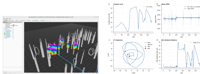
图 11: 场景 4 静态避障: RViz (左) 与评测曲线 (右)
