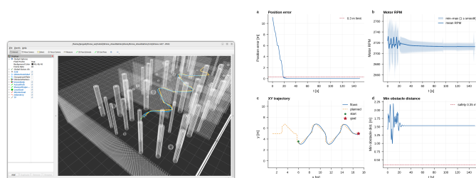
图 12: 场景 5 窄通道: RViz (左) 与评测曲线 (右)
