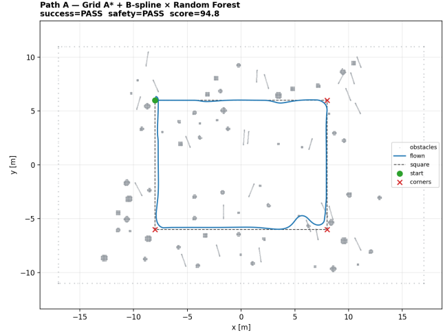
图 16: Path A 森林试次轨迹
