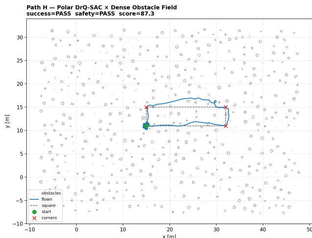
图 19: Path H 密集场试次轨迹
