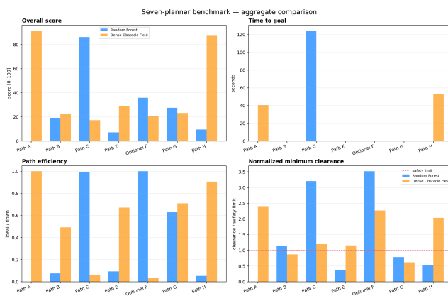
图 14: 规划器对照总览图
