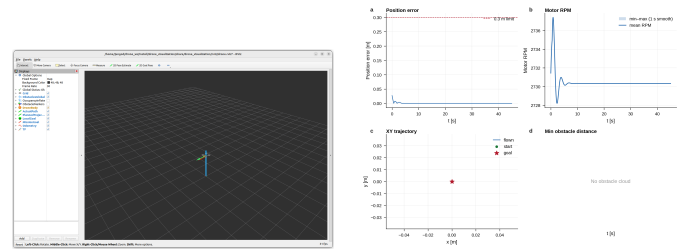
图 8：场景 1 悬停：RViz（左）与评测曲线（右）
