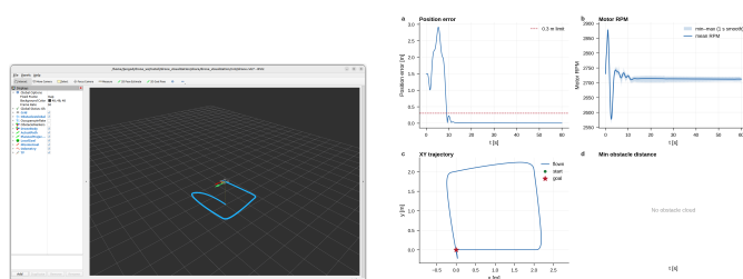
图 10: 场景 3 多航点: RViz (左) 与评测曲线 (右)
