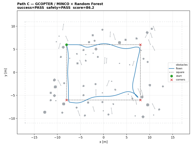
图 17: Path C 森林试次轨迹
