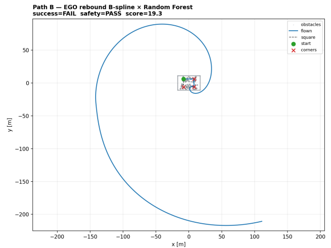
图 18: Path B 森林试次轨迹
