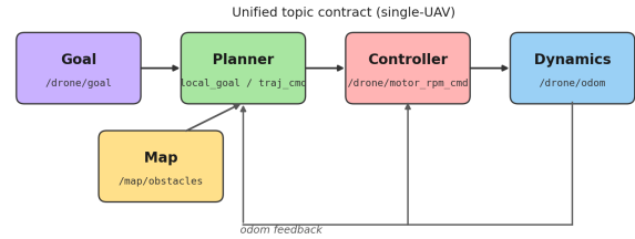
图 2：单机统一话题契约与状态反馈
