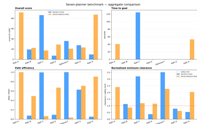
图 14: 规划器对照总览图
