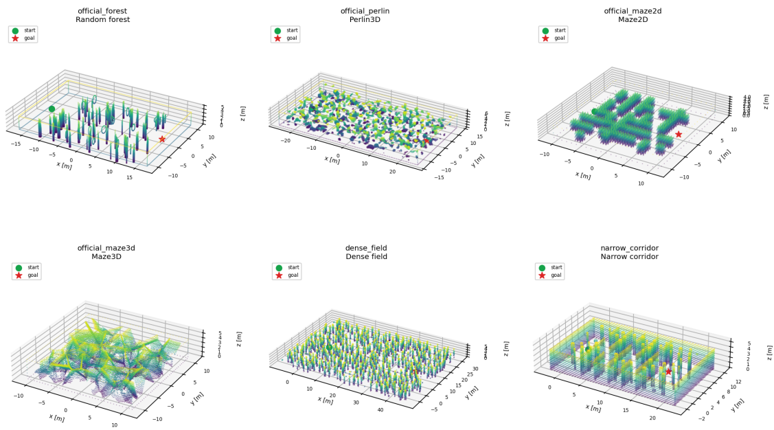
图 3：主要仿真地图三维斜视点云（两行 × 三列）。颜色表示高度；绿点为起点，红星为目标。
