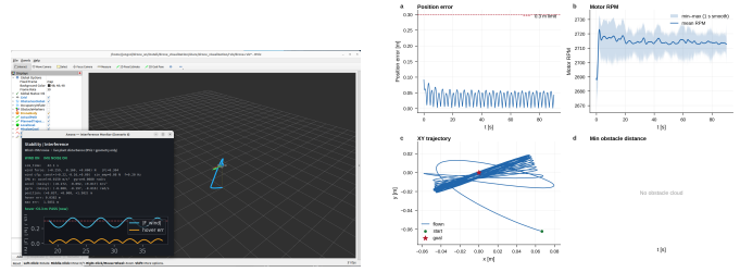
图 13: 场景 6 稳定性: RViz (左) 与评测曲线 (右)
