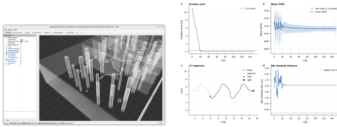
图 12: 场景 5 窄通道: RViz (左) 与评测曲线 (右)
