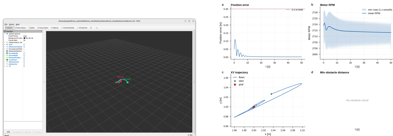
图 5: 场景 2 单目标: RViz (左) 与评测曲线 (右)
