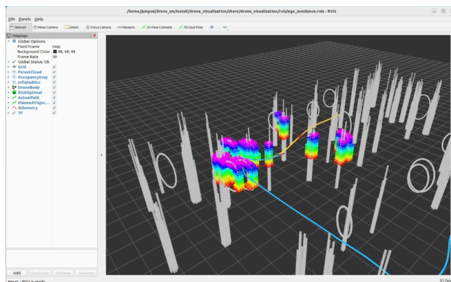
图 7: 场景 4 静态避障: RViz (左) 与评测曲线 (右)
