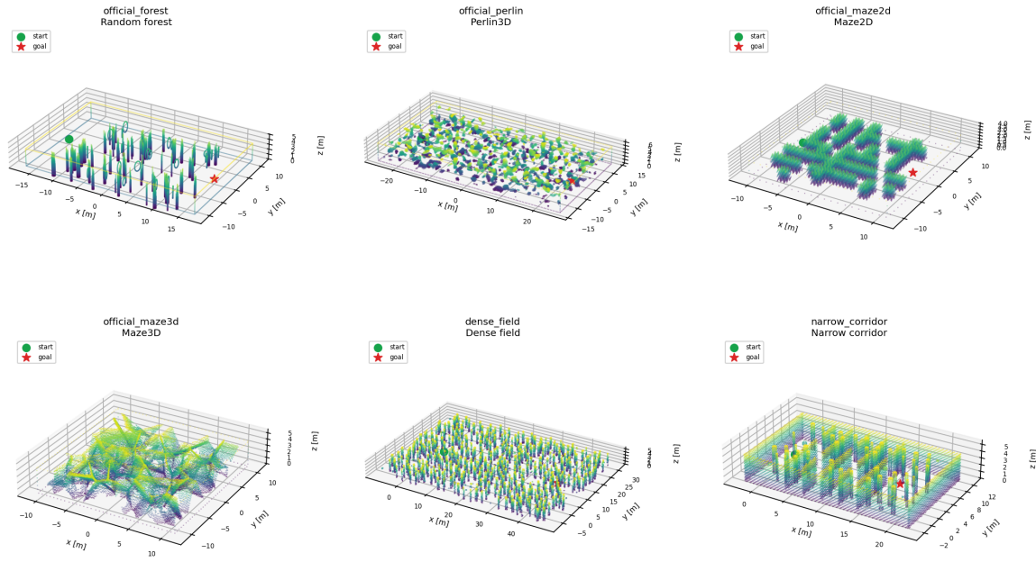
图 10：主要仿真地图三维斜视点云。颜色表示高度；绿点为起点，红星为目标。
