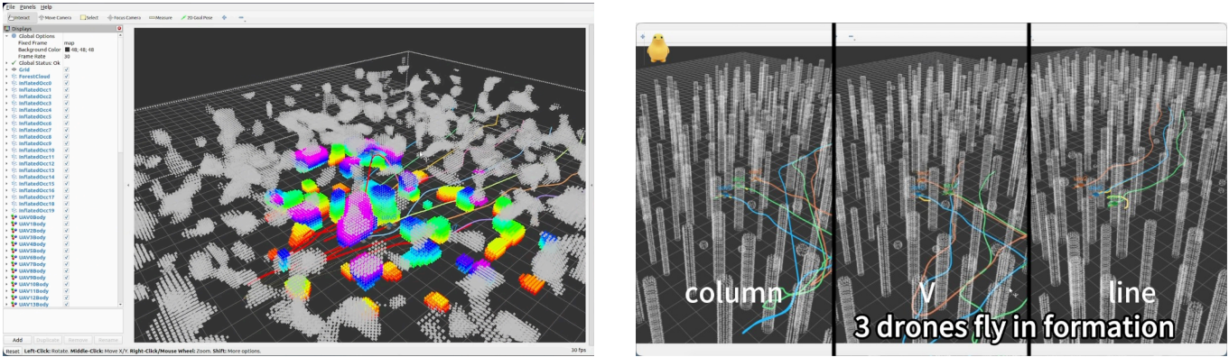
图 12：左：八机 Ego-Swarm 协同；右：三机编队（column / V / line）
