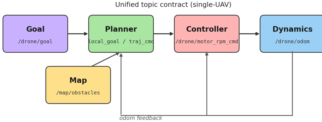
图 2: 单机统一话题契约与状态反馈
