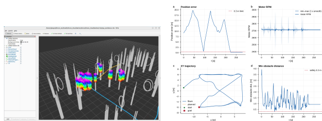
图 7: 场景 4 静态避障: RViz (左) 与评测曲线 (右)
