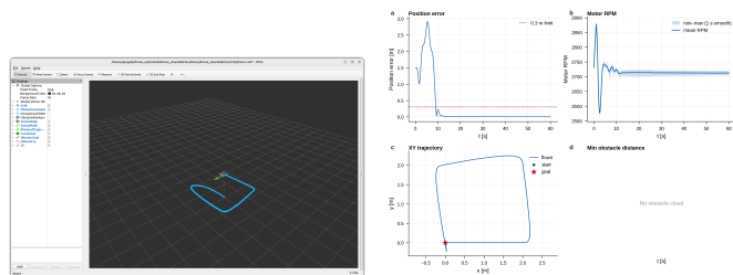
图 6: 场景 3 多航点: RViz (左) 与评测曲线 (右)
