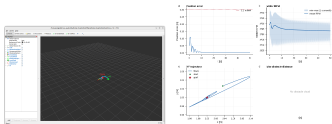
图 5: 场景 2 单目标: RViz (左) 与评测曲线 (右)
