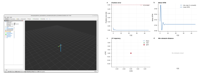
图 4: 场景 1 悬停: RViz (左) 与评测曲线 (右)
