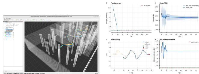
图 8: 场景 5 窄通道: RViz (左) 与评测曲线 (右)
