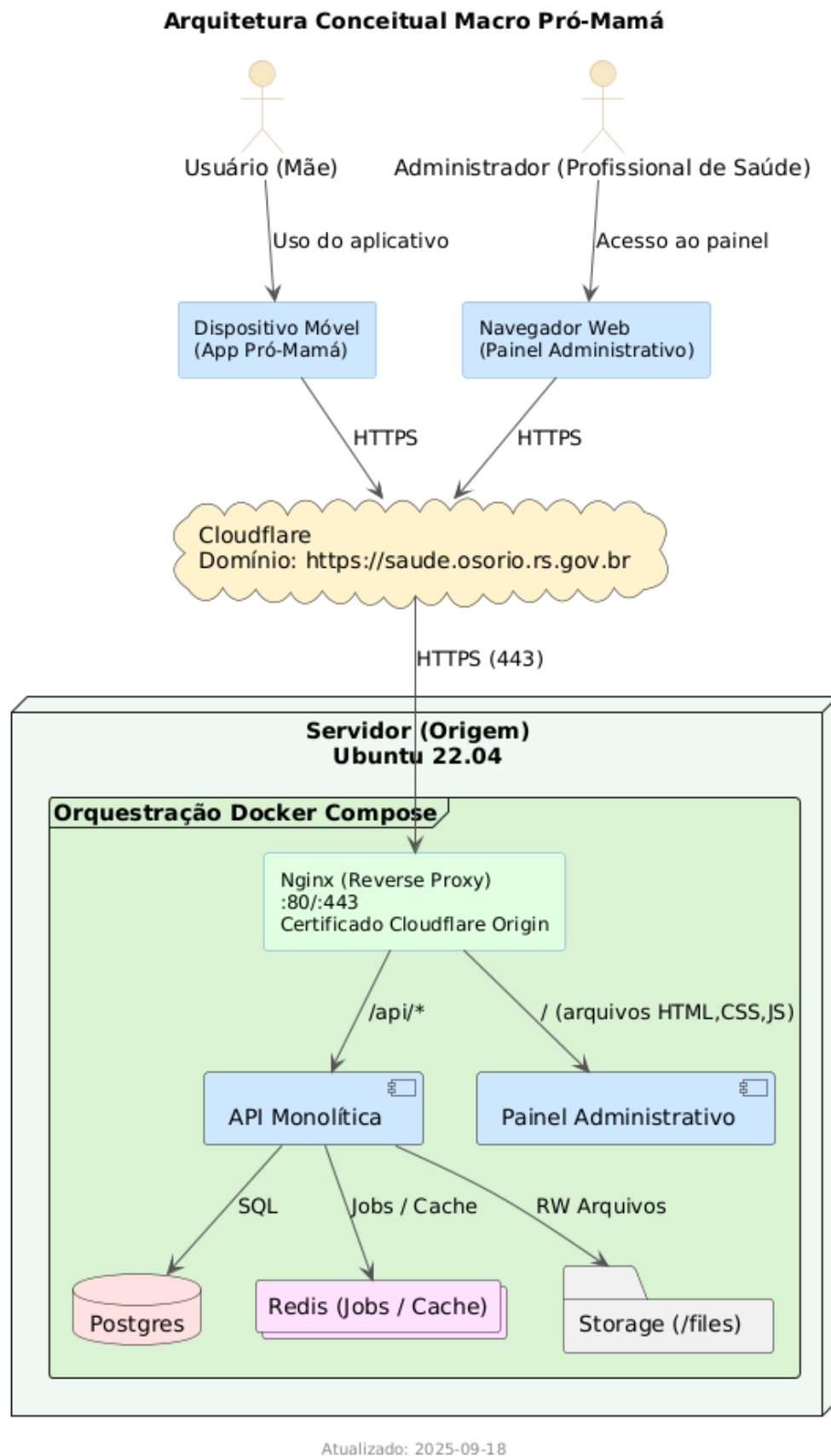
Figura 3 – Visão geral dos componentes e interações do sistema Pró-Mamá. Fonte: Autoria Própria.
