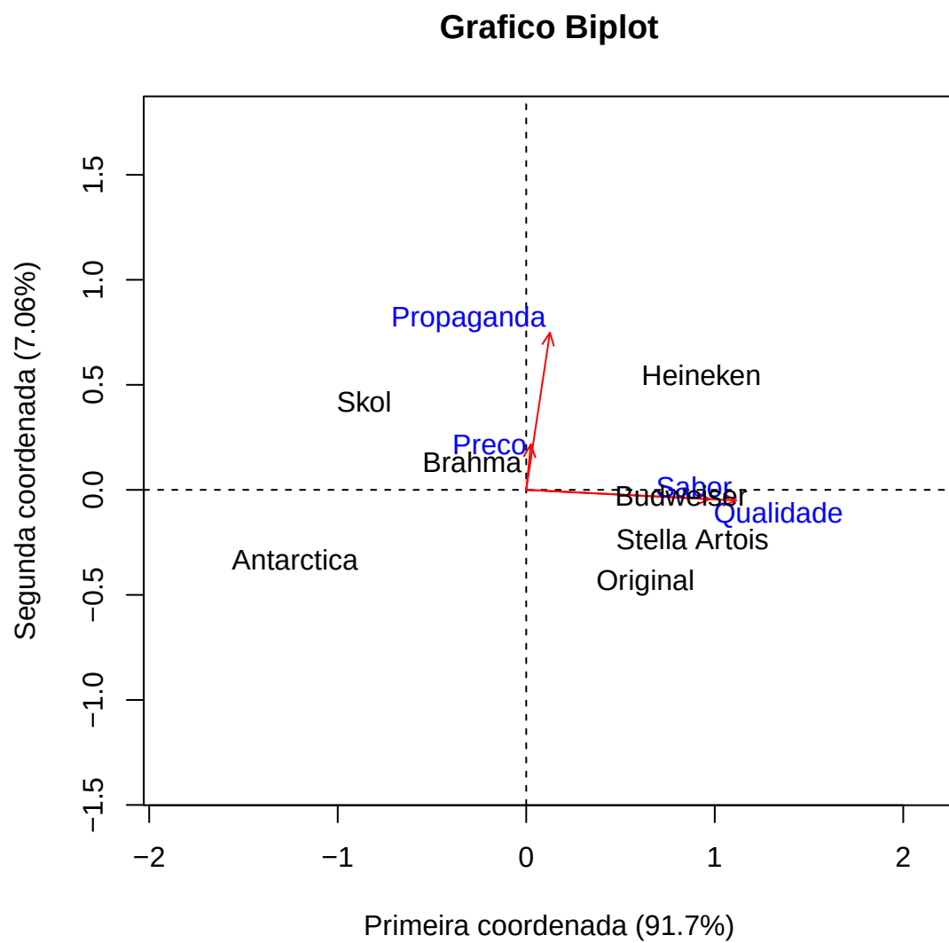
Figura 2: Biplot EM
