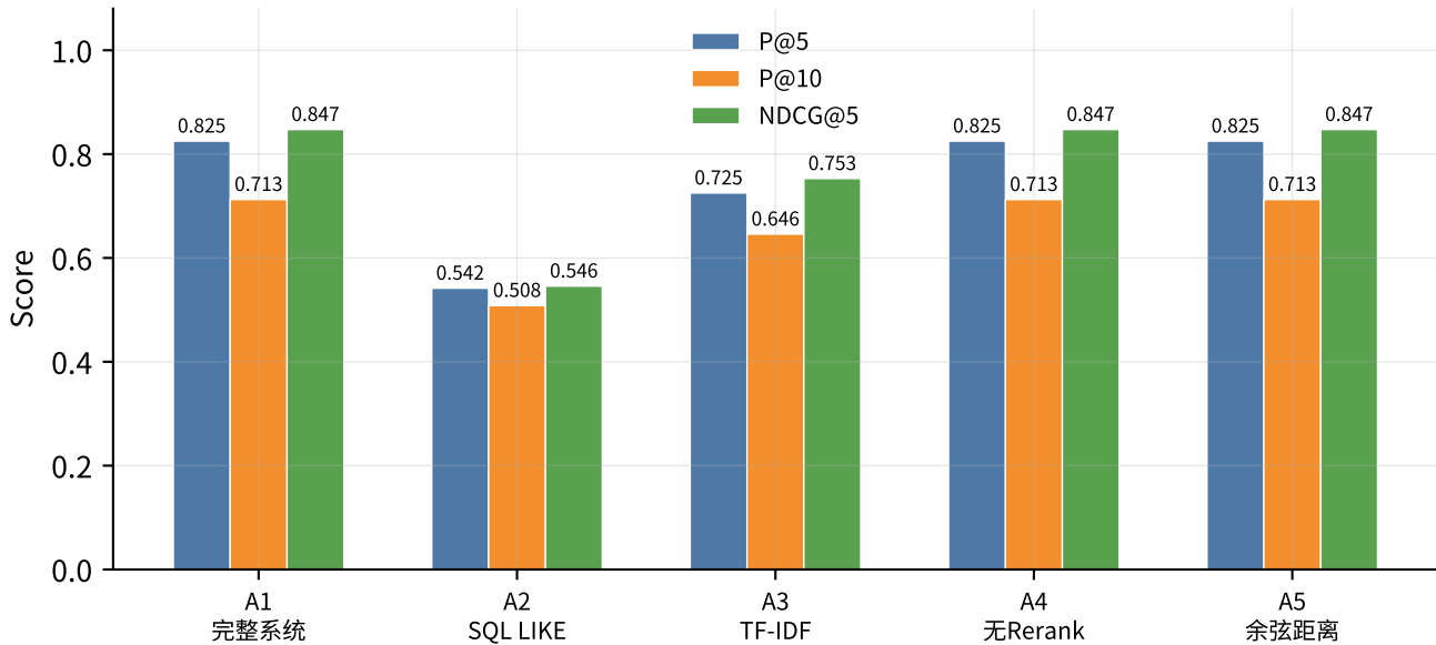
搜索系统消融实验
