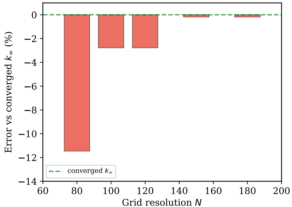
(b) Error vs k_{\infty}
