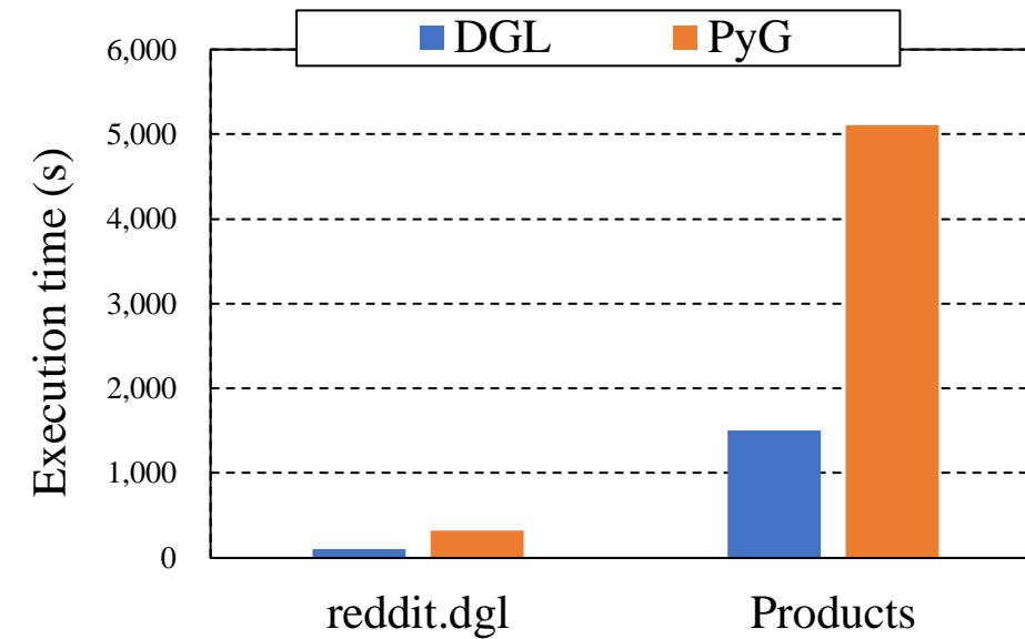
GCN
