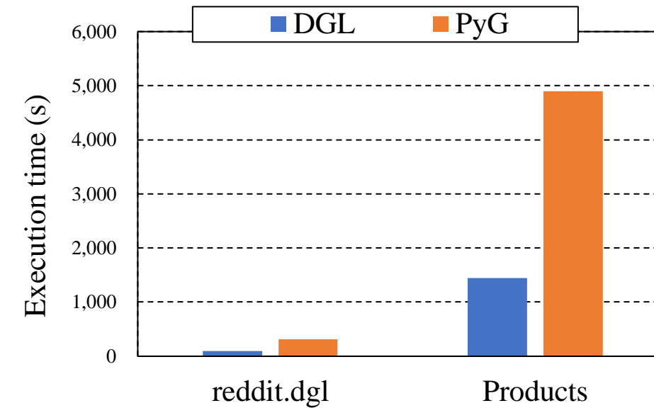
GIN
