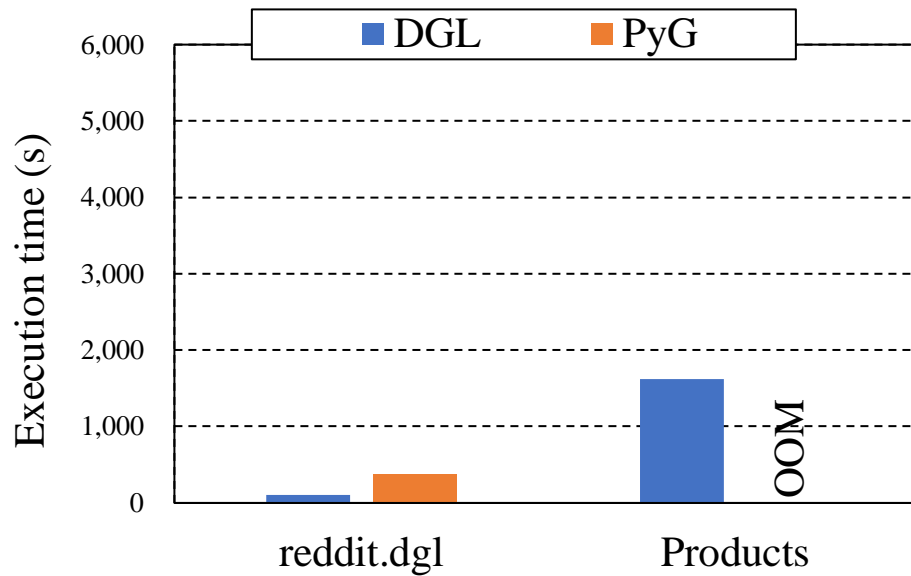
GAT
