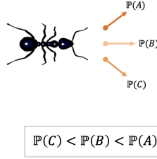
Figura 3.6: Possíveis movimentos da formiga P(x) , [12].
