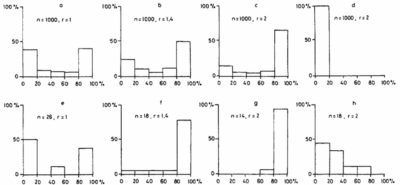
Figura 2.2: Resultados da experiência de Goss et al [3].
